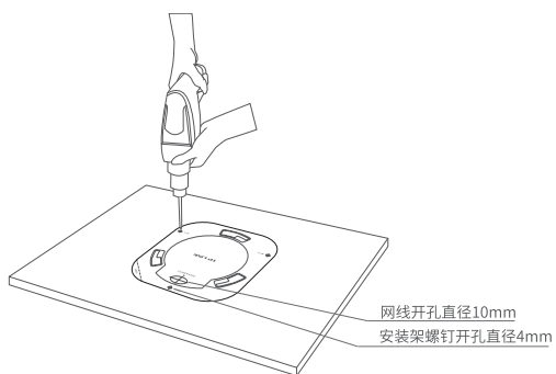
图3-3 钻孔示意图
